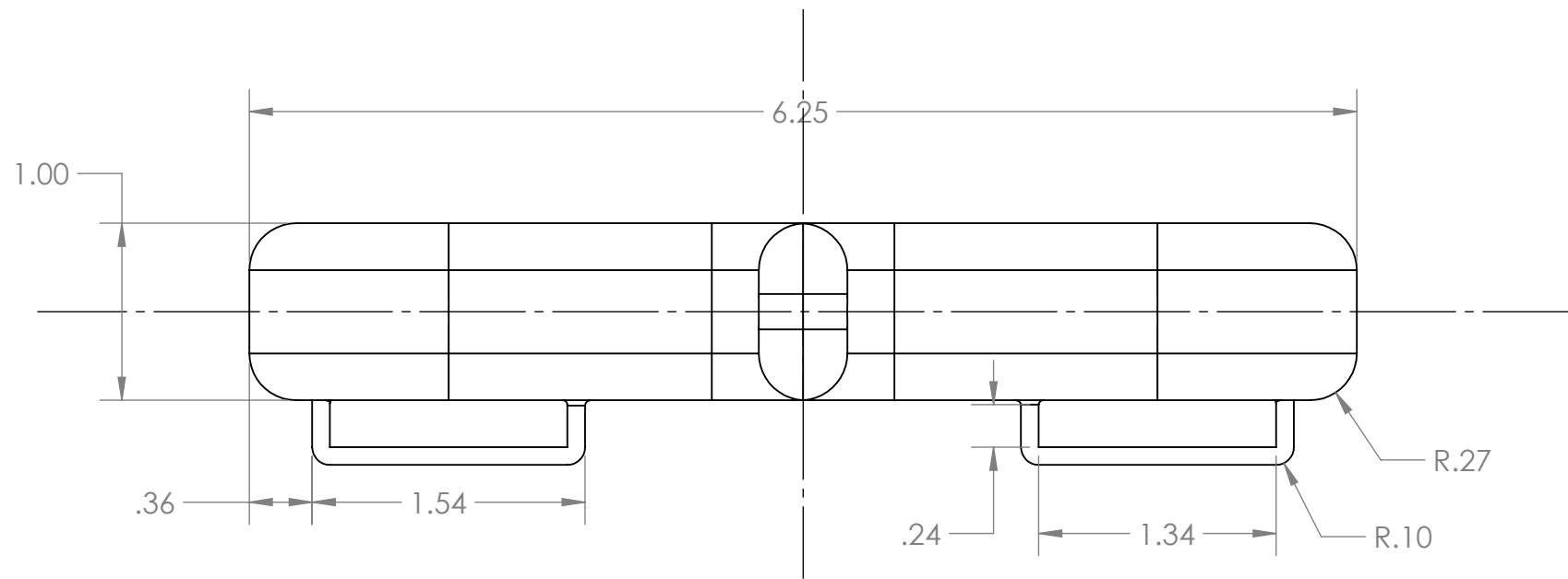
TOP
