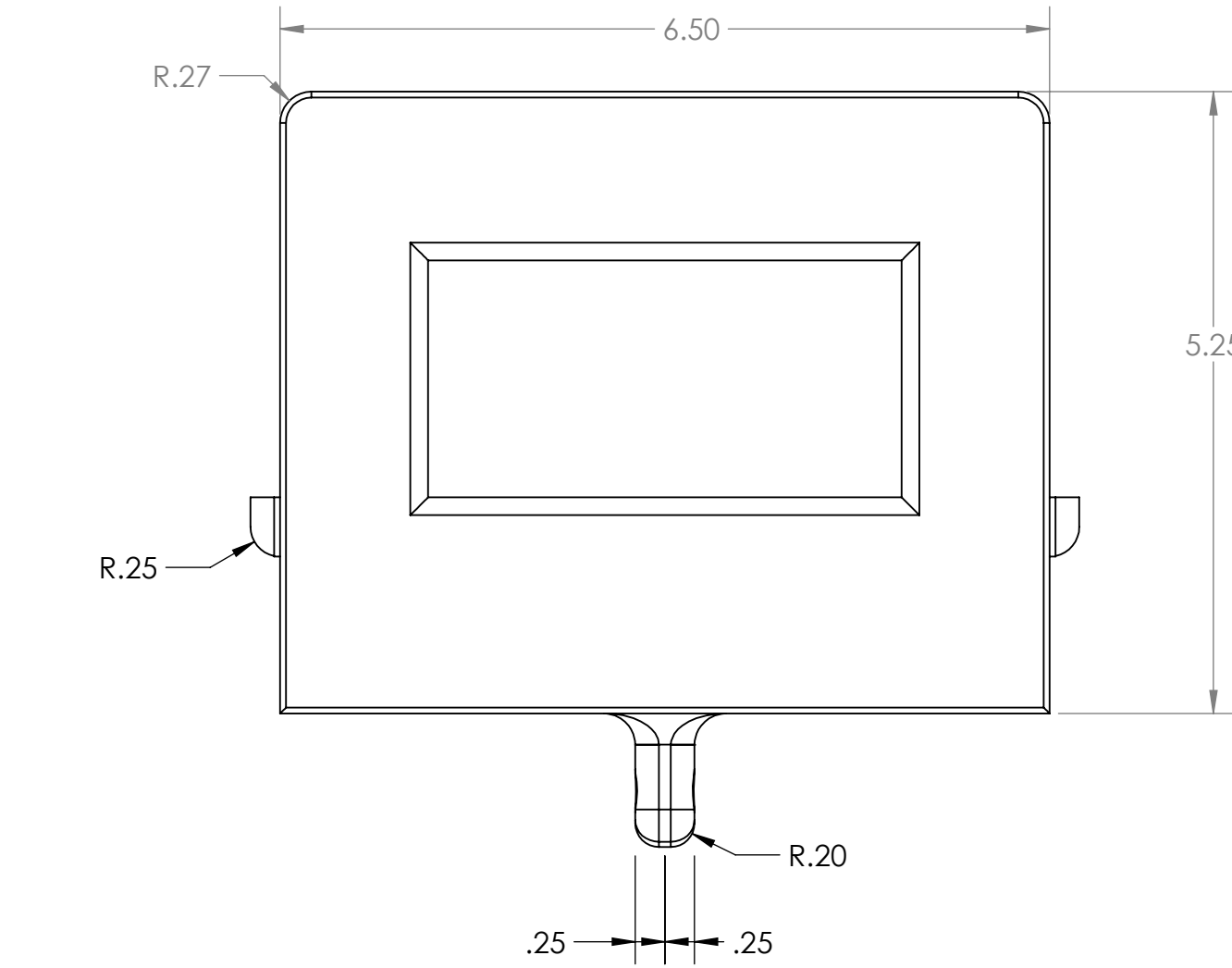
TOP
