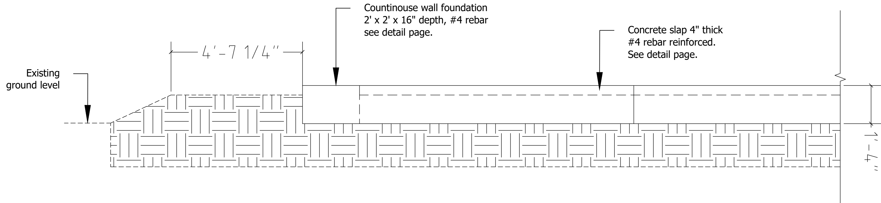
Detail SCALE: 3/8"=1' 0"
